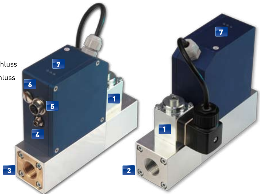
Rückseite des flox[on] B economy und extended
